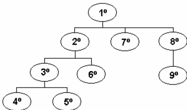
Orden de recorrido de un árbol en preorden
