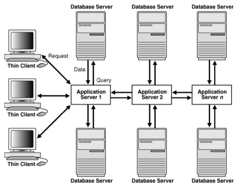
Arquitectura multitier .
